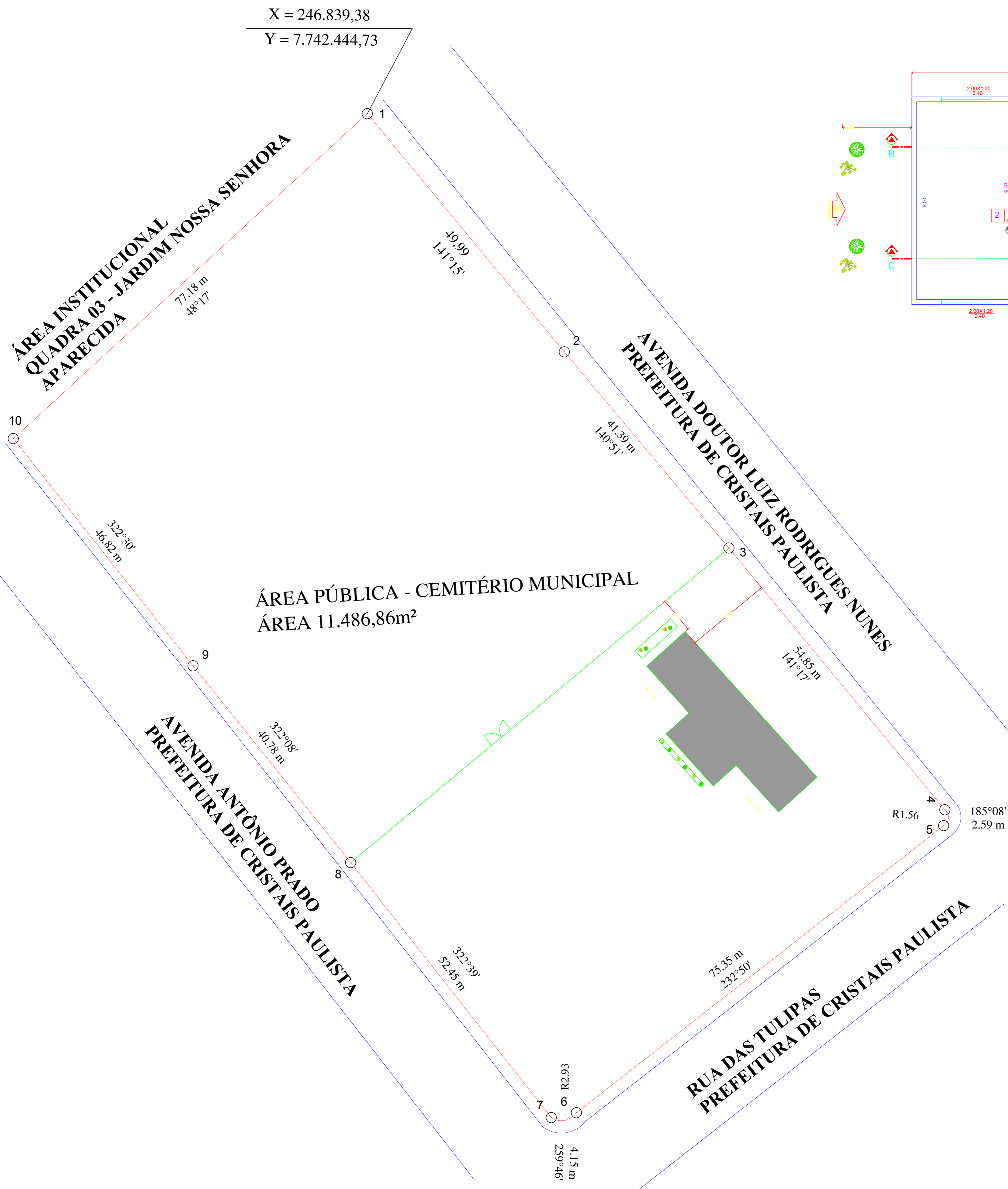
PLANTA DE IMPLANTAÇÃO Escala 1:200
